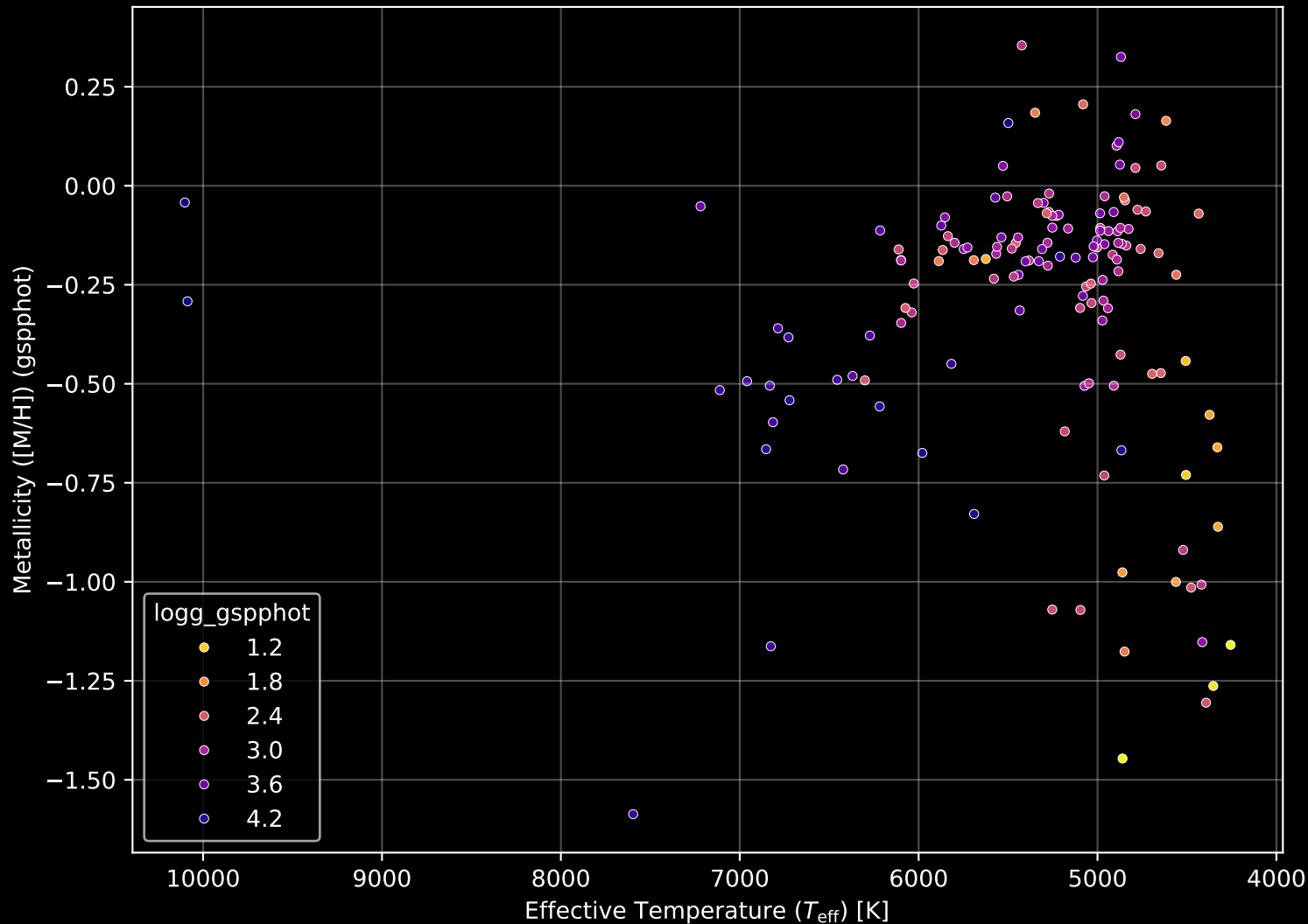
APOGEE DR17 Field: [000+30] Stellar Population Parameters (n= 147)
